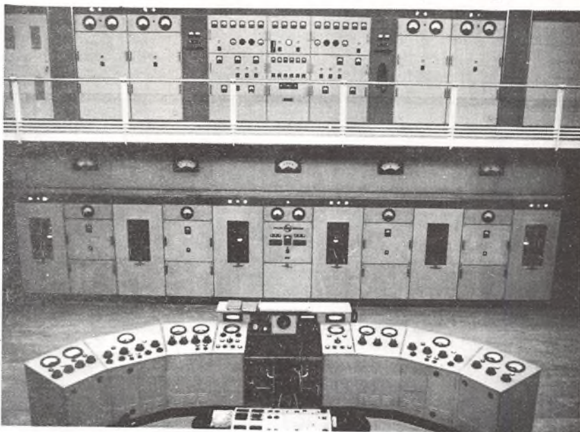
Nieuwe middengolffzender 600 kW.
