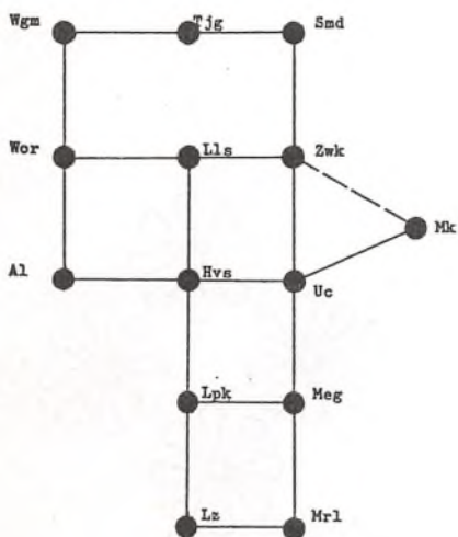
Schematische weergave routing van het koppelnet.
