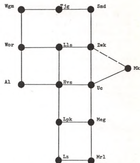
Schematische weergave routing van het koppelnet
