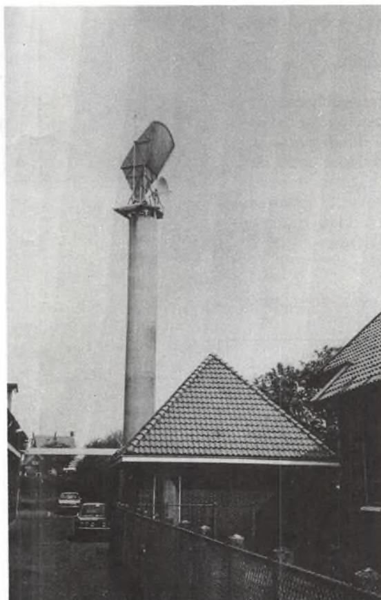
De straalverbindingsmast met de parabolantennes gericht op Goes
